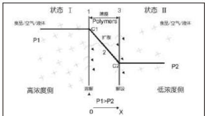
图一 渗透过程原理图
