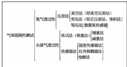
图二 气体阻隔性的测试方法与原理
